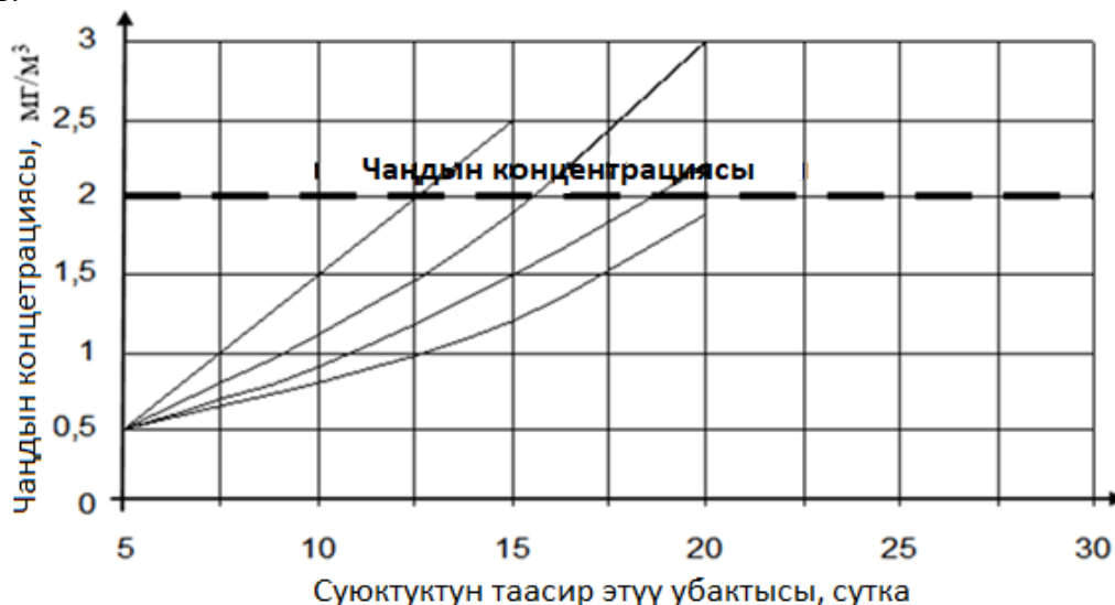
12-сүрөт – Технологиялык автожолду сугаргандан кийинки чанды басуу натыйжалуулугу [12]:
