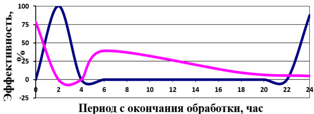
11-сүрөт – Технологиялык карьердик автожолдордо чаңды басуунун натыйжалуулугу [11-13]: 1 – суу; 2 - ПАА
