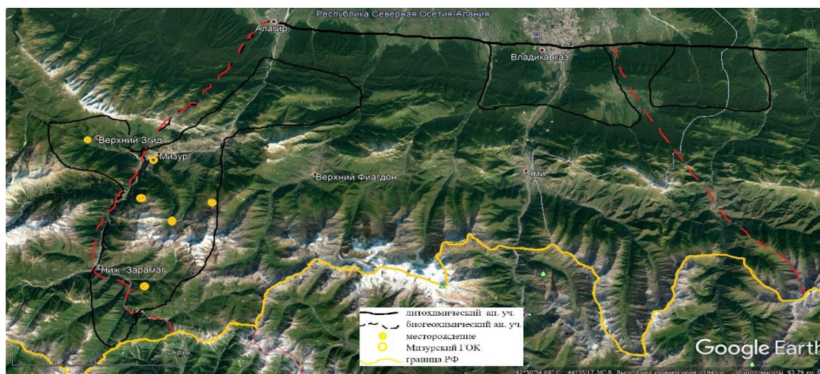
6-сүрөт - Садон кенинен тартып химиялык элементтерин таралышы
