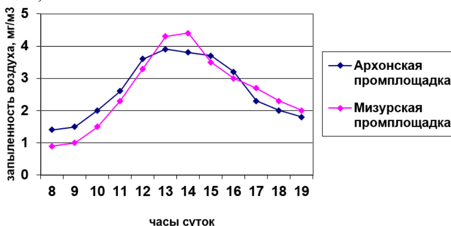
3-сүрөт –Күндүз атмосферанын жердеги катмарындагы абанын чаңдашы
